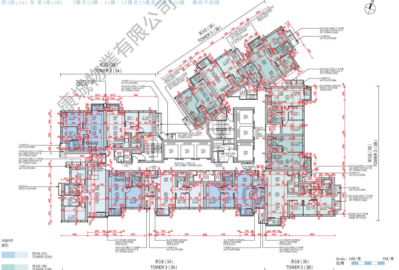
Tower 3(3A) & Tower 3(3B) 第3座(3A)及第3座(3B) 7/F-12/F, 15/F, 17/F-23/F & 25/F-26/F 7樓至12樓、15樓、17樓至23樓及25樓至26樓 Floor Plan 樓面平面圖
